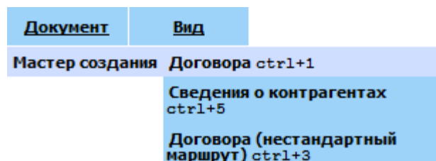
Рисунок 5. Создание документа
