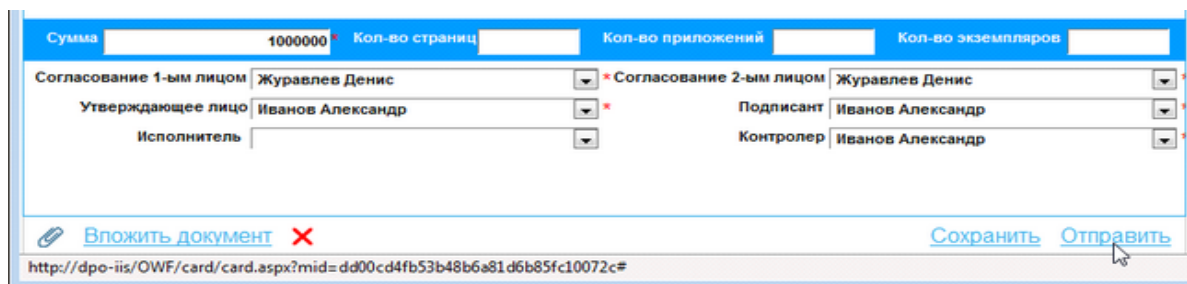
Рисунок 14. Отправка документа
